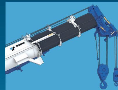
伸縮モード2 [3段目・4段目・トップブーム先伸長方式]
