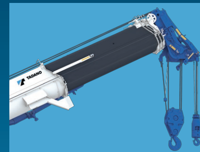
伸縮モード1 [2段目ブーム先伸長方式]
